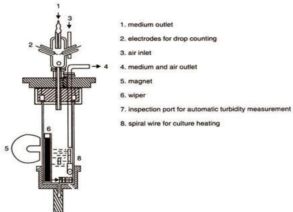
Fig. 2.13: Turbidostat
